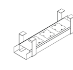
插座线槽 DT-T01-S W400 x D120 x H110
