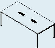
DT-MT Conference Table 会议台 W1600 x D800 x H745 W1800 x D900 x H745 W2000 x D1000 x H745 W2200/2400 x D1100 x H745
