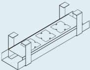
插座线槽 DT-T01-S W400 x D120 x H110
