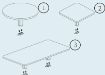
多功能架 ① ASC-30 Φ30 x H20 ② ASS-30 W30 x D30 x H20 ③ ASR-3060 W60 x D30 x H20
