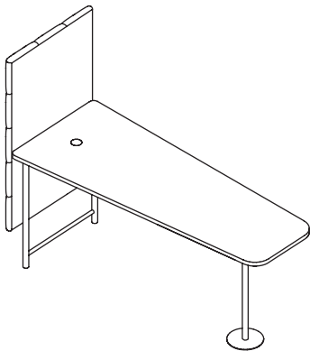
Meeting Table / 会议台 Three seaters / 三座位 PUFF-MT-03-HF W680 x D1700 x H1360 mm
