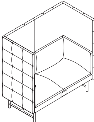
Two seaters / 双座位 PUFF-SF-02-HFHK (香港插座制式) PUFF-SF-02-HFCN (中国插座制式) W1390 x D695 x H1360 mm
