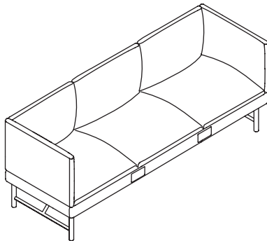
Three seaters / 三座位 PUFF-SF-03-FHK (香港插座制式) PUFF-SF-03-FCN (中国插座制式) W1950 x D650 x H750 mm
