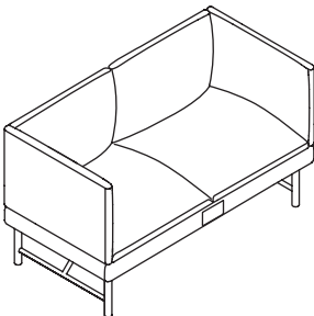
Two seaters / 双座位 PUFF-SF-02-FHK (香港插座制式) PUFF-SF-02-FCN (中国插座制式) W1300 x D650 x H750 mm
