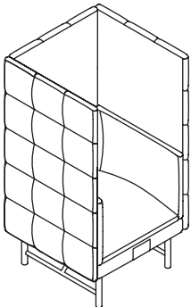
One seater / 单座位 PUFF-SF-01-HFHK (香港插座制式) PUFF-SF-01-HFCN (中国插座制式) W740 x D695 x H1360 mm
